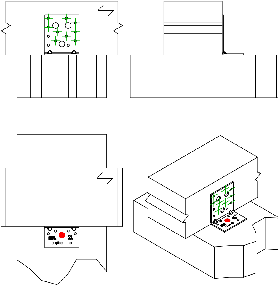
Montering med 1 beslag
