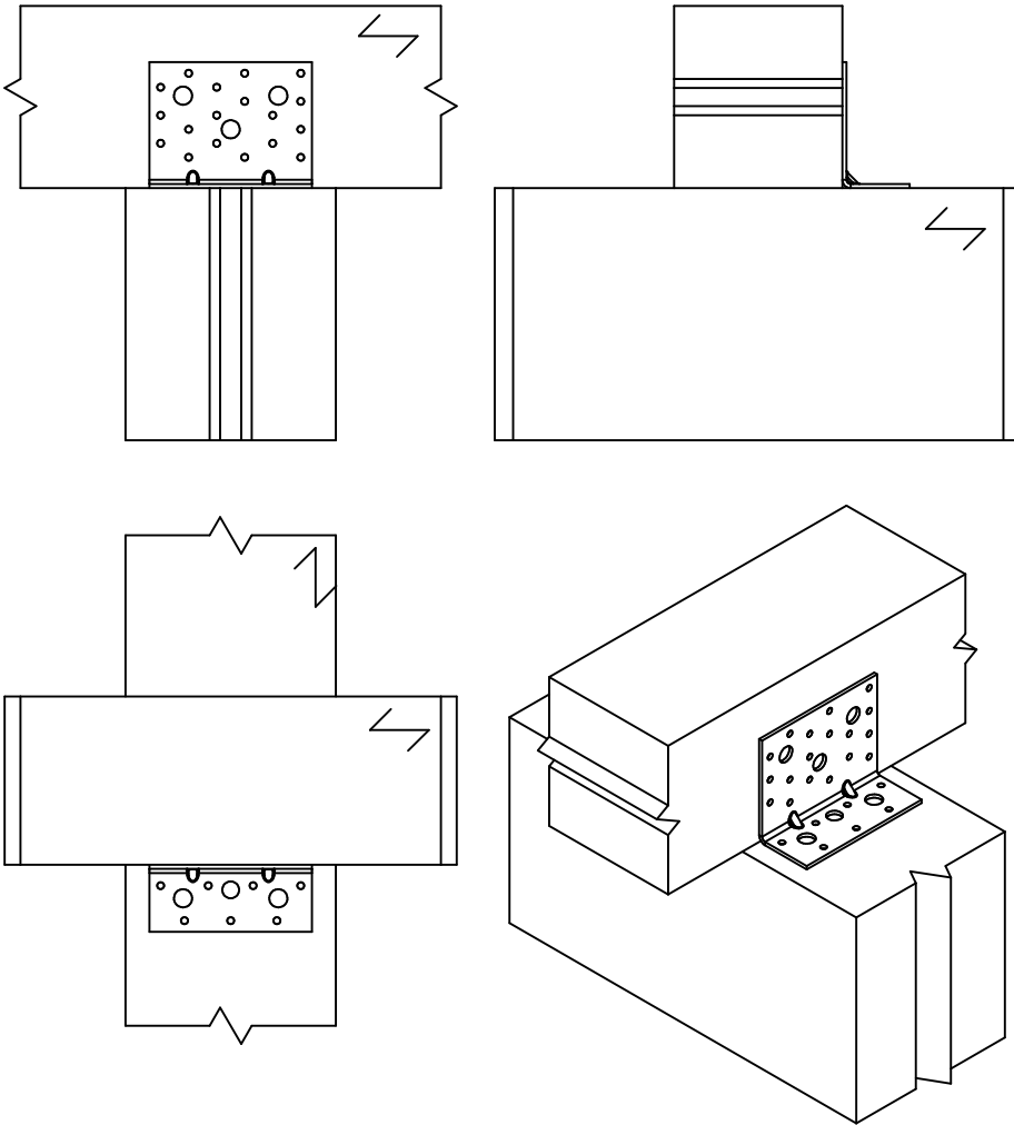
Einbau bei 1 Winkel
